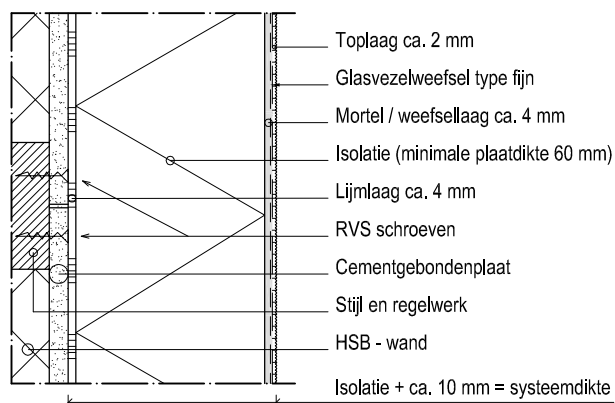
STRIKOTHERM COMFORT - DECORATIEVE SIERPLEISTER OP HSB-WAND
